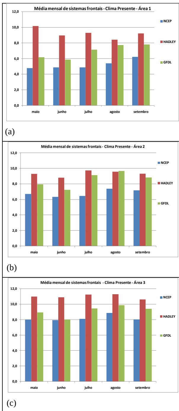
Figura 2: Média mensal de sistemas frontais nas áreas (a) 1; (b) 2 e (c) 3 para o NCEP, GFDL e Hadley para o clima presente.
