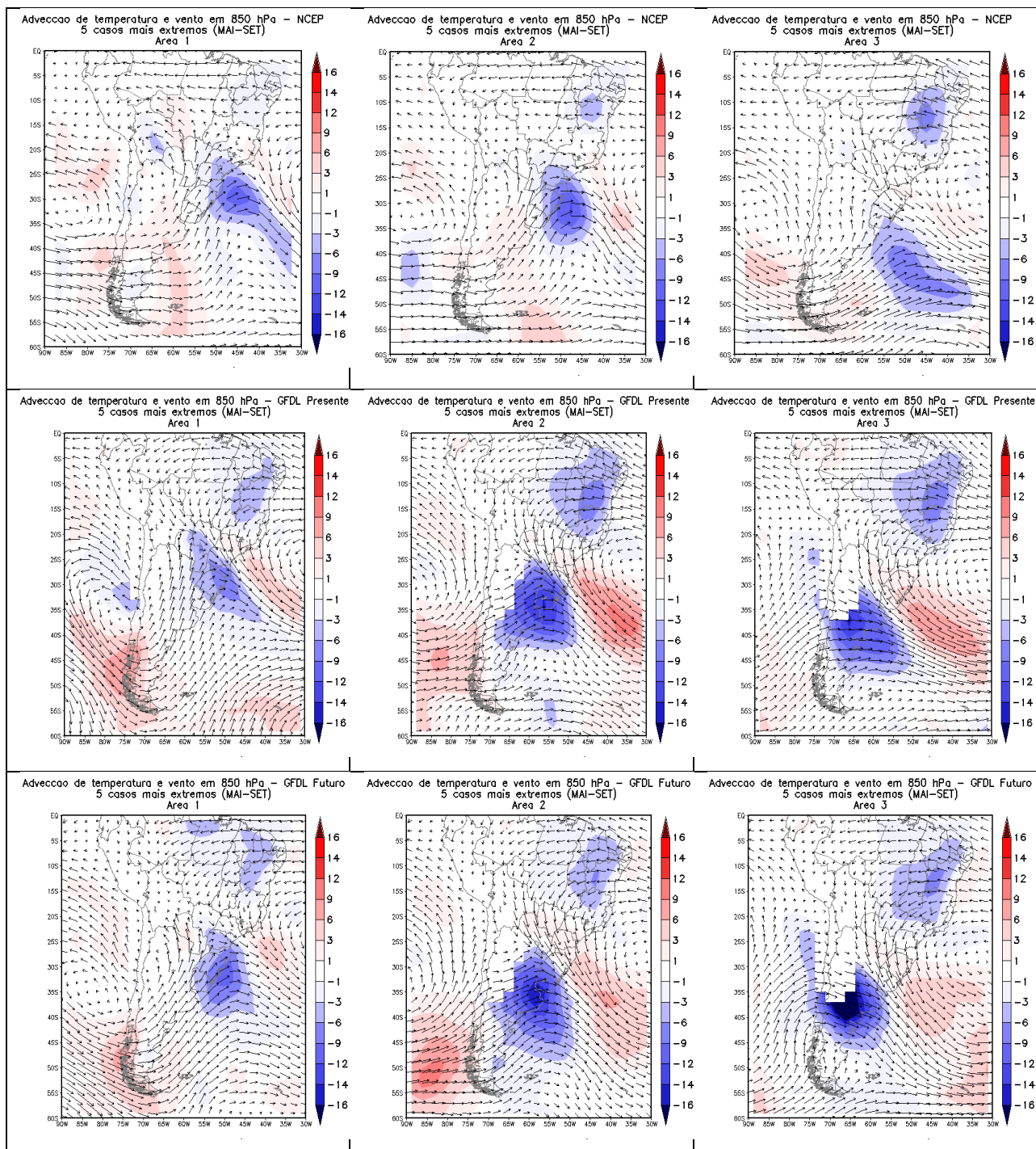
Figura 7: Advecção de temperatura ( ^{\circ}\text{C}/\text{dia} ) e vetor vento ( \text{m/s} ) em 850 hPa: área 1 (primeira coluna), área 2 (segunda coluna), área 3 (terceira coluna) para reanálise (primeira linha; GFDL presente (segunda linha); GFDL-Futuro (terceira linha)).
