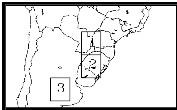
Figura 1: Áreas com as três regiões utilizadas na determinação das frentes
