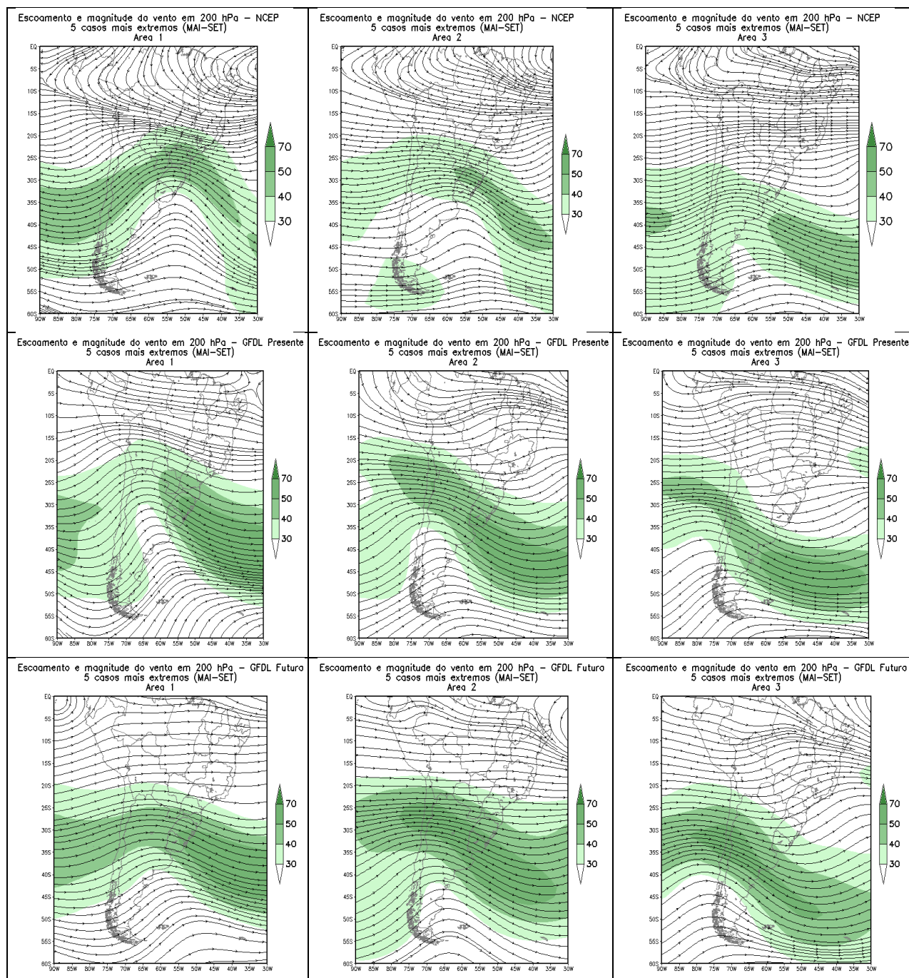
Figura 8: Escoamento e magnitude do vento (m/s) em 200 hPa: área 1 (primeira coluna), área 2 (segunda coluna), área 3 (terceira coluna) para reanálise (primeira linha; GFDL presente (segunda linha); GFDL-Futuro (terceira linha)).
