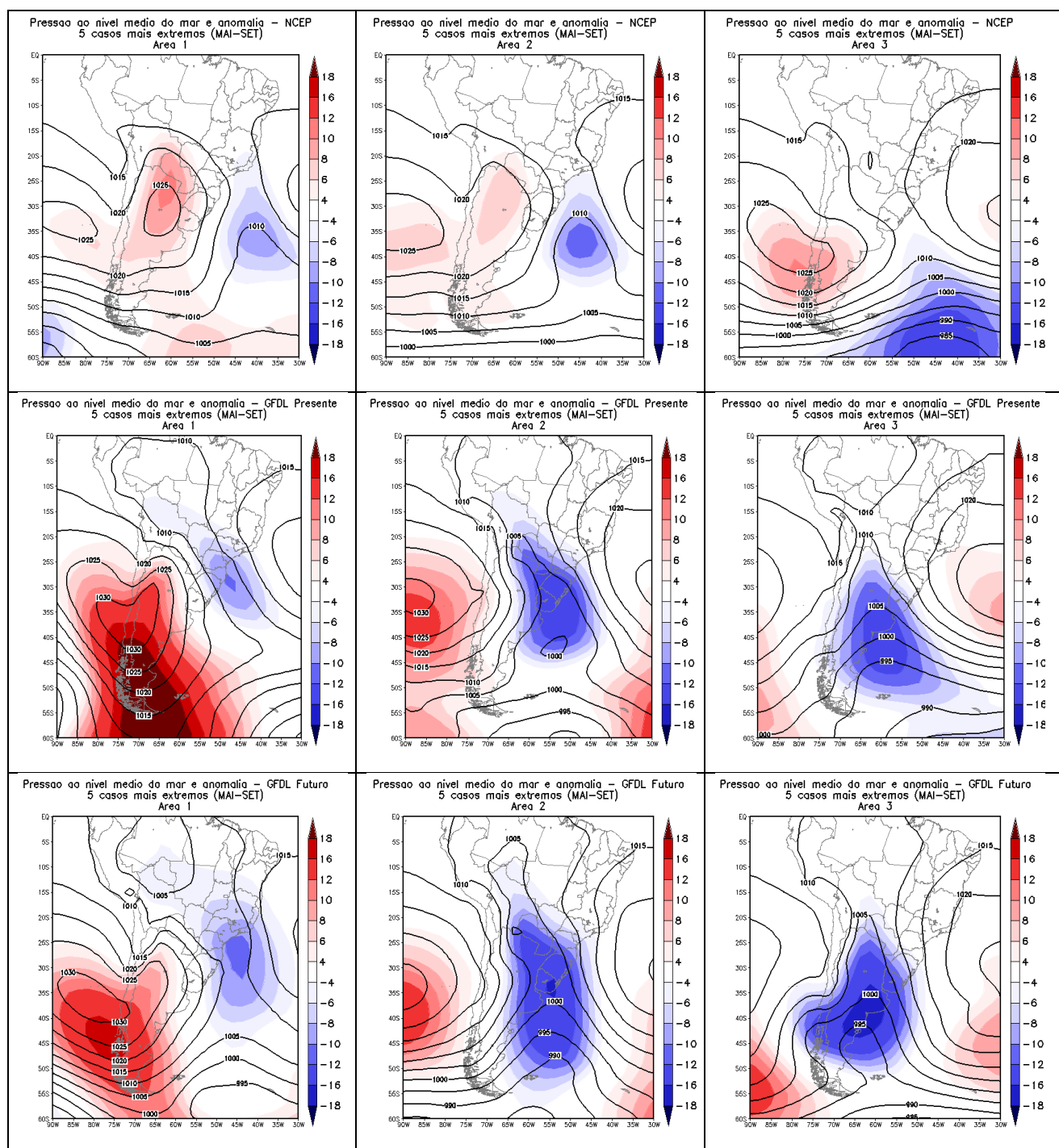
Figura 6: Pressão ao nível médio do mar e anomalia (hPa): área 1 (primeira coluna), área 2 (segunda coluna), área 3 (terceira coluna) para reanálise (primeira linha); GFDL presente (segunda linha); GFDL-Futuro (terceira linha).
