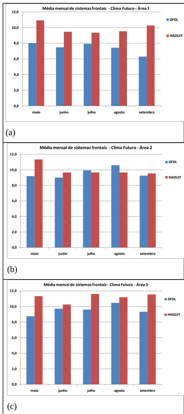
Figura 4: Média mensal de sistemas frontais nas áreas (a) 1; (b) 2 e (c) 3 para o GFDL e Hadley para o clima futuro.
