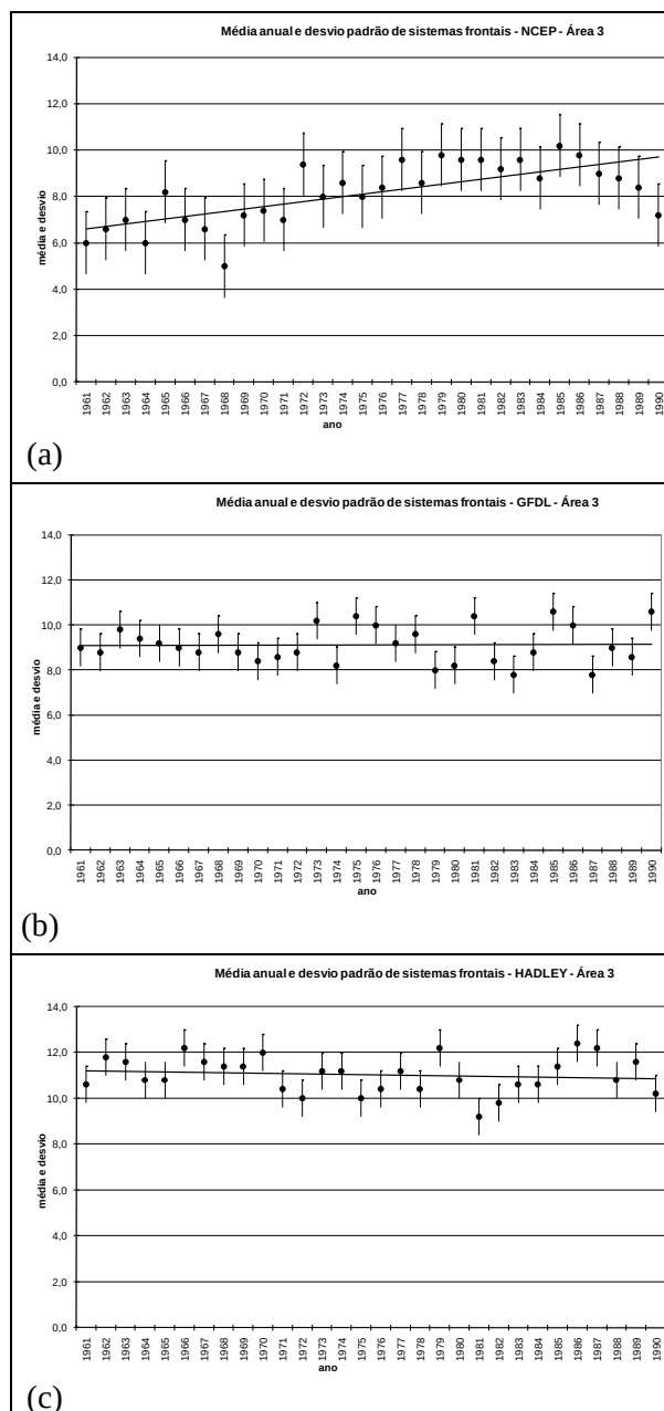
Figura 3: Média de sistemas frontais e desvio padrão para o período de maio a setembro de cada ano (em número/mês) para (a) NCEP (b) GFDL (c) Hadley na área 3 no período entre 1961-1990.
