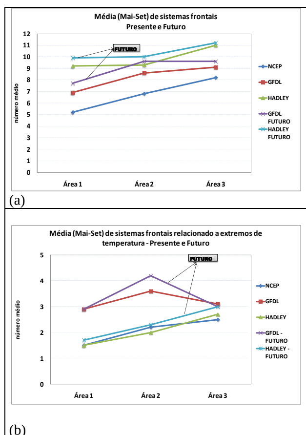
Figura 5: (a) Média do número de sistemas frontais no período entre maio e setembro ( n^\circ/\text{mês} ) no clima presente e futuro. (b) Mesmo que em (a), mas para os casos extremos de temperatura.
