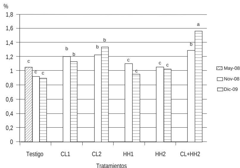
FIGURA 2. Evolución del carbono orgánico particulado (COP). Diferentes letras muestran diferencias significativas (Fisher p < 0,05 ).
