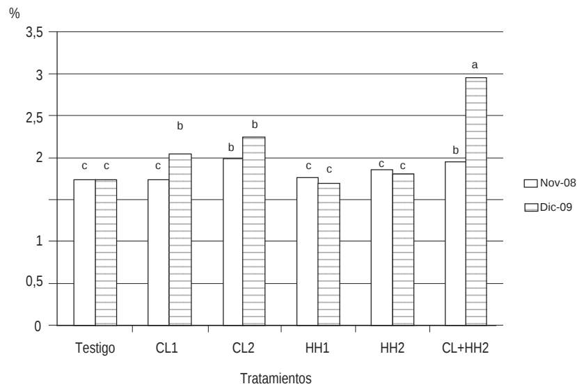
FIGURA 3. Evolución de la relación AH/AF. Diferentes letras muestran diferencias significativas (Fisher p < 0,05 ).
