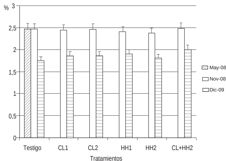
FIGURA 1. Evolución del carbono oxidable. Diferentes letras muestran diferencias significativas (Fisher p < 0,05 ).
