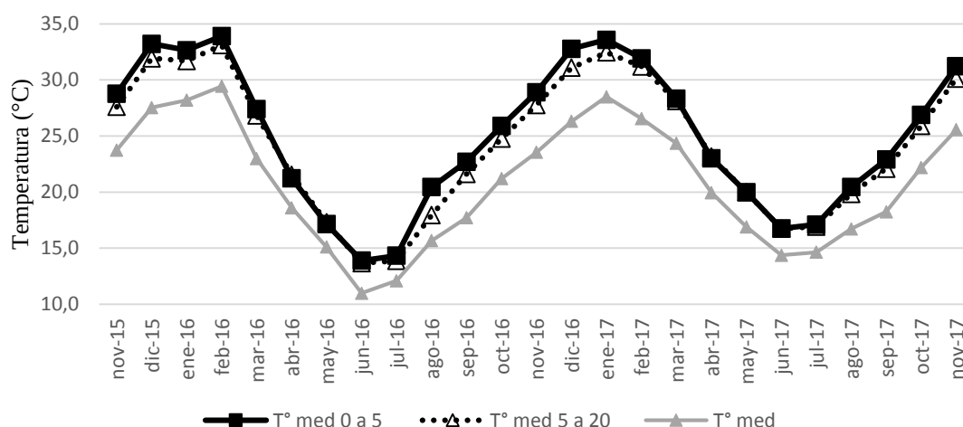
Figura 1.4. Temperatura media mensual del suelo de 0 a 5 cm y de 5 a 20 cm para el período noviembre de 2015 - noviembre de 2017. Temperatura media mensual ( T^{\circ} med); Temperatura media mensual de suelo en la profundidad de 0 a 5 cm, expresada en °C ( T^{\circ} med 0 a 5); Temperatura media mensual de suelo en la profundidad de 5 a 20 cm, expresada en °C ( T^{\circ} med 5 a 20). (Registros de estación agrometeorológica automática del INTA Santiago del Estero).
