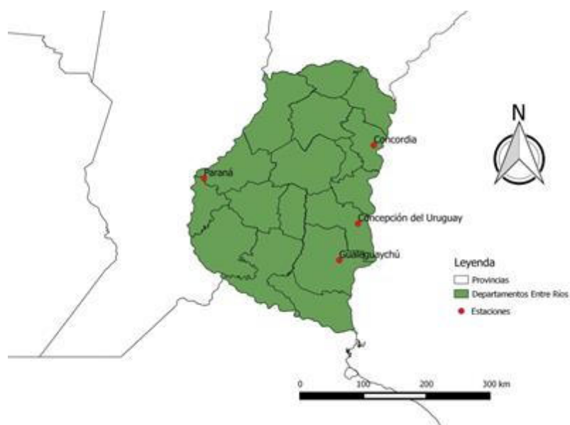
Figura 2.1. Localización de las EMC utilizadas para generar precipitaciones interpoladas departamentales y SPI.
