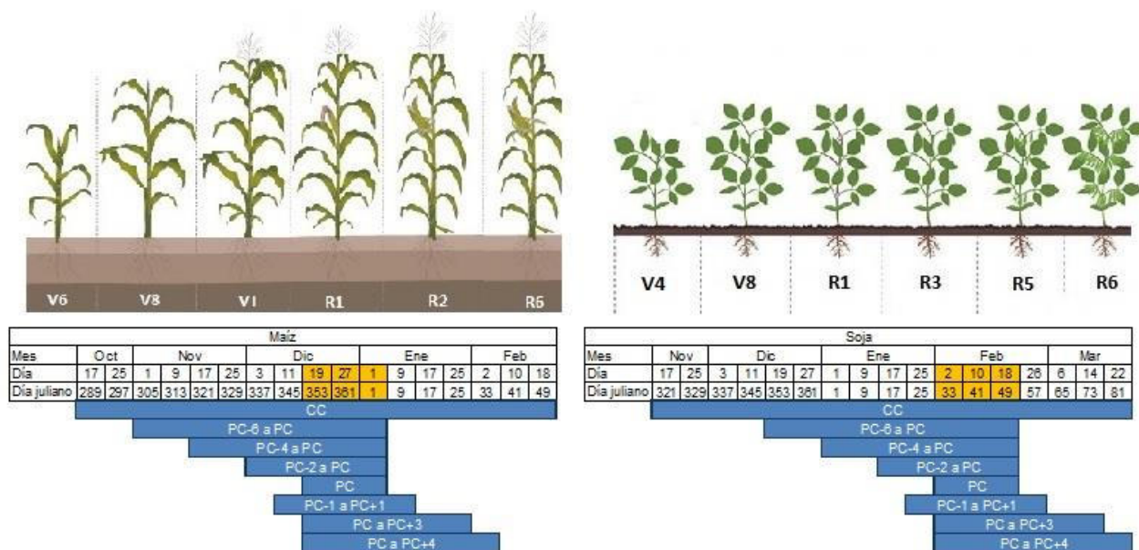
Figura 4.2. Períodos (bloques azules) en los que se promedió cada índice escalado y VHI para correlacionar con el rendimiento final del cultivo y estadios fenológicos aproximados. Referencias: CC = ciclo completo, PC = período crítico (fecha marcada en color anaranjado), PC-n o PC+n = n indica el número de fechas previas consideradas (en períodos de 8 días) antes (-) o después (+) del PC.
