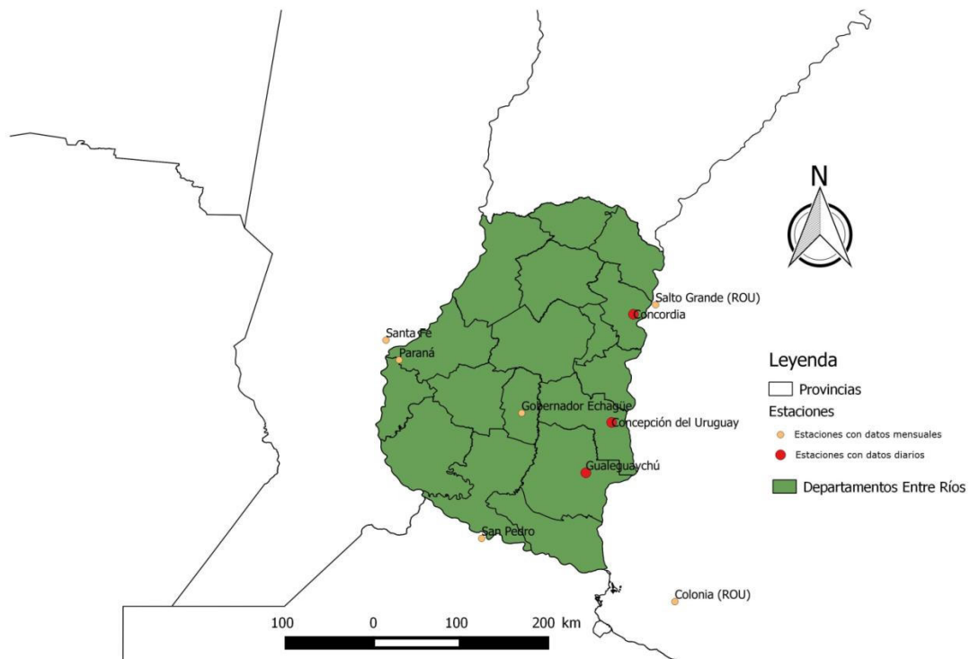
Figura 3.1. Mapa con la ubicación de las EMC utilizadas para evaluar la capacidad de TRMM de estimar precipitaciones mensuales y de distintos períodos de acumulación en Entre Ríos.
