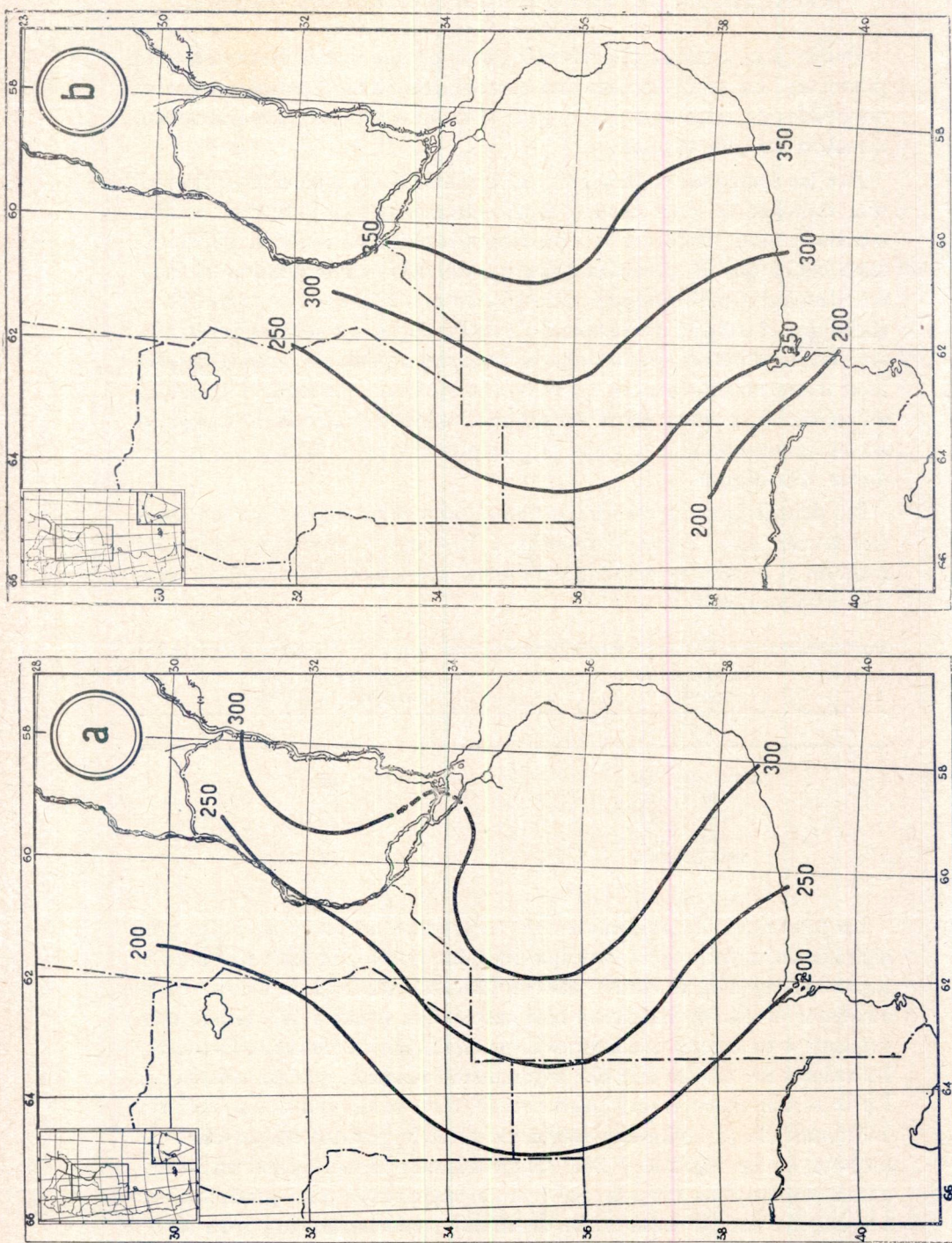
Fig. 28. — Disponibilidad de agua (milímetros) durante el período siembra-maduración. a ) y b ) Precipitación media para los trigos semiprecoces y semitardíos, respectivamente.
