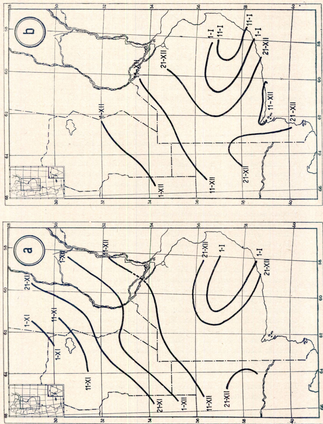
Fig. 23. — Isofenas de cosecha. a) Trigos semiprecoces. b) Trigos semitardíos
