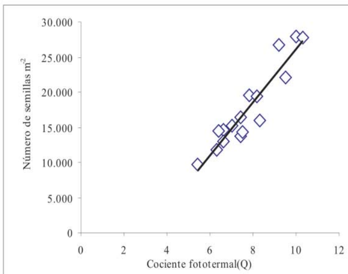
FIGURA 10. Relación entre el número de semillas \text{m}^{-2} y cociente fotothermal (Q) para los tratamientos S1, S2, S3, S4 y S5, en los años 2000, 2001, 2002 y 2003 ( y = 3787,1x - 11687 ; r^2 = 0,88 ), calculado para los 20 días previos a antesis y los 10 días posteriores.
