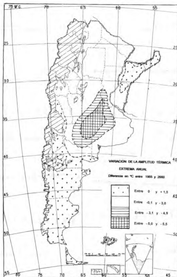
Figura 2. Variación de la amplitud térmica extrema anual en el período 1965-2000.
