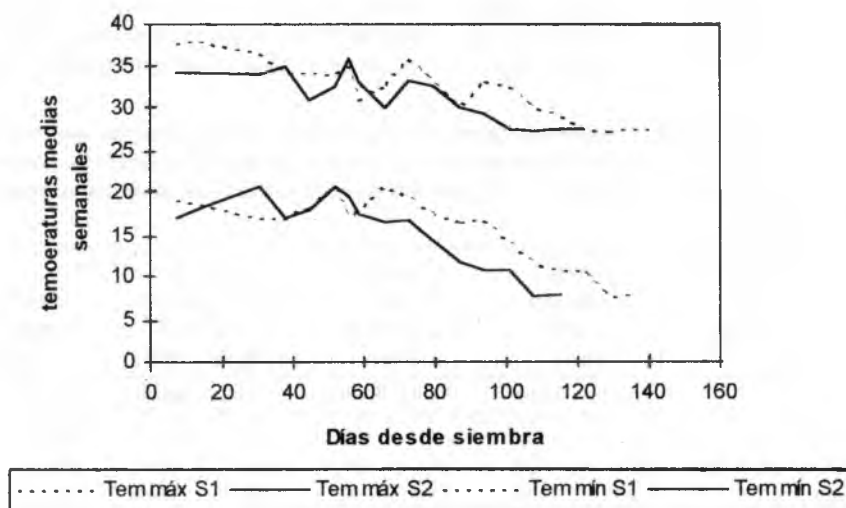
Figura 1. Temperaturas mínimas y máximas medias semanales registradas por el cultivo desde siembra hasta el 01/05/96. S 1 : 22-12-95 y S 2 : 12-01-96
