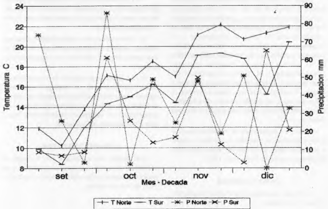
Figura 1: Temperatura y precipitación decadica Zona Norte-Sur. Periodo anual: 1990 Fuente: Ing. Agr. R. Maschini. (Climatología y Meteorología Agrícola, INTA-Castelar)
