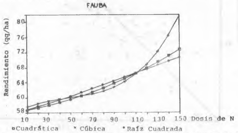
Figura 3: Rendimiento predicho por distintas formas algebraicas en función de la dosis de N. Datos de FAUBA.
