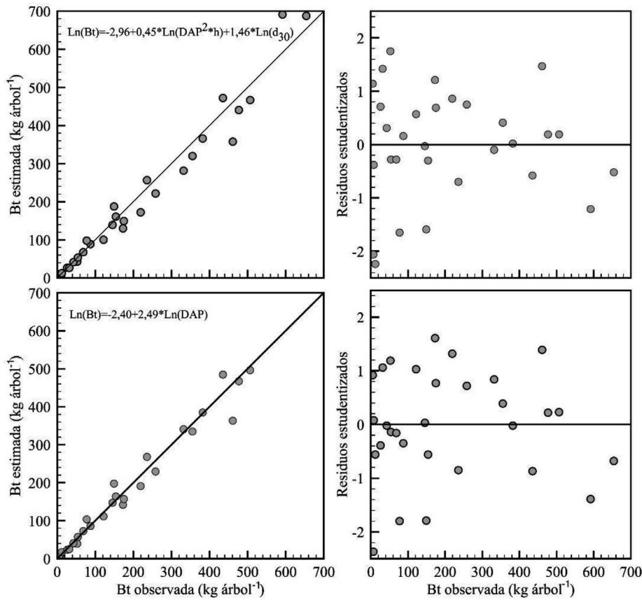
Figura 2. Ecuaciones alométricas de biomasa aérea total de individuos de Prosopis nigra basados en DAP^{2 \times h} y d_{30} , y en DAP (izquierda), con sus correspondientes gráficos de residuos (a la derecha). Cada punto representa una observación individual ( n=30 ). Bt: biomasa aérea total ( \text{kg árbol}^{-1} ); DAP: diámetro a la altura del pecho (cm); h: altura total (m); d_{30} : diámetro basal a 0,30 m desde el nivel del suelo (cm).
