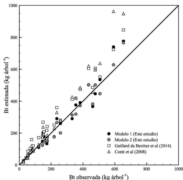
Figura 3. Comparación entre las estimaciones de biomasa total (Bt) en Prosopis nigra obtenidas a partir de diferentes modelos. Se muestra la biomasa estimada ( \text{kg árbol}^{-1} ) vs. la observada ( \text{kg árbol}^{-1} ), a partir de 4 modelos: Modelo 1 (este estudio): \text{Ln (Bt)} = -2,96 + 0,45 \cdot \text{Ln (DAP}^2 \cdot h) + 1,46 \cdot \text{Ln (d}_{30}) ; Modelo 2 (este estudio): \text{Ln (Bt)} = -2,40 + 2,49 \cdot \text{Ln (DAP)} ; Gaillard de Benítez et al. (2014): \text{Bt} = -97,97 + 6,28 \cdot \text{DAP} + 0,49 \cdot \text{DAP}^2 ; Conti et al. (2008): V = 0,05 \cdot d_{15}^{2,78} , siendo V: volumen aéreo ( \text{dm}^3 ).
