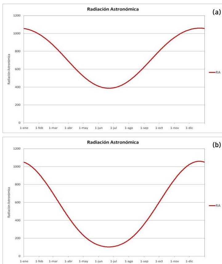
Figura 5. Radiación astronómica diaria (RA) en \text{cal/cm}^2\text{min} para Pergamino (a) y Ushuaia (b).
