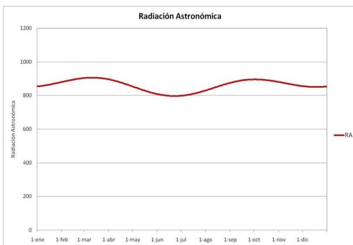
Figura 6. Radiación astronómica diaria (RA) en \text{cal/cm}^2\text{min} sobre el Ecuador.
