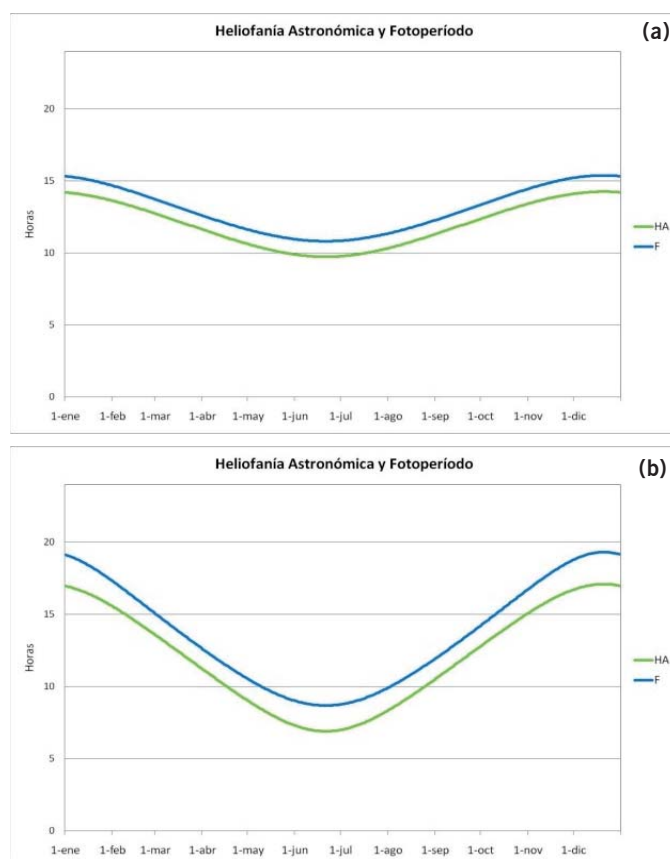
Figura 4. Heliofanía astronómica (HA) y fotoperíodo (F) para Pergamino (a) y Usuhaia (b).
