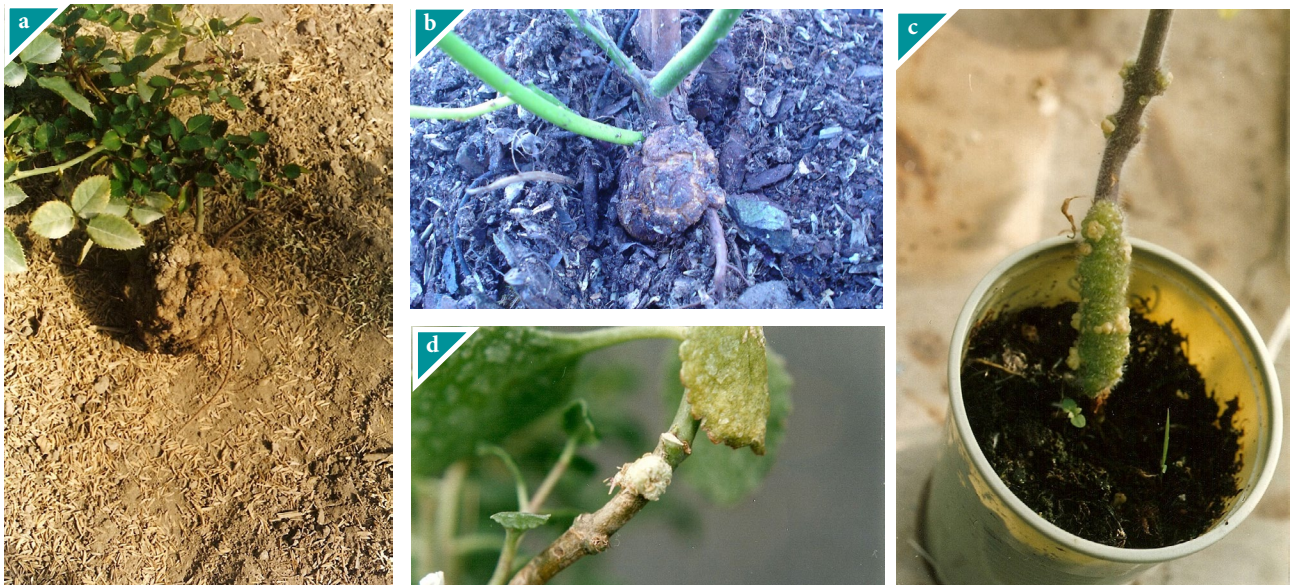
Figura 13.18. Agalla de corona, sintomatología: a.b. agallas leñosas basales en rosal y arándano, c.d. agallas carnosas aéreas en plantas de tomate y kalanchoe inoculadas.
