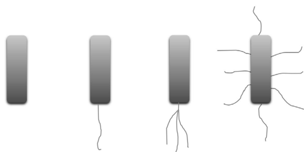
Figura 7.2. Denominación de las células bacterianas según la disposición de los flagelos. De izquierda a derecha: aflagelada, monótrica, lofótrica, perítrica.
