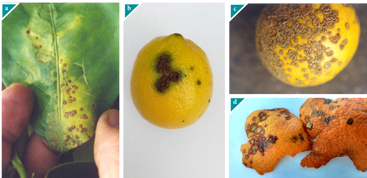
Figura 13.16. Cancrosis de los cítricos, sintomatología: a. erupciones corchosas en hojas, b.c.d. erupciones corchosas en superficie de limón, pomelo y mandarina.
