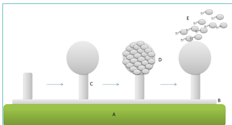
Figura 6.8. Formación de una zoospora . A= hospedante, B= hifa no tabicada, C= zoosporangióforo, D= zoosporangio, E= zoospora.
