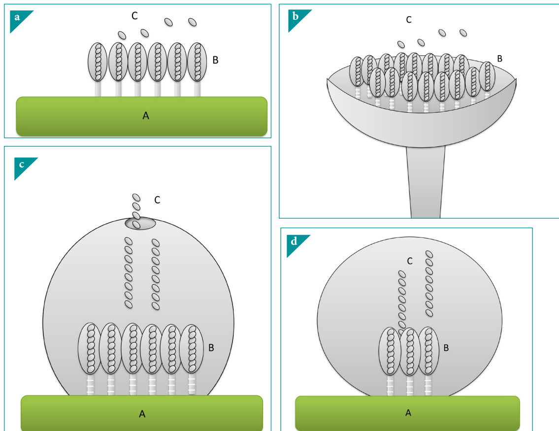
Figura 6.12. a. Ascos libres. b. Ascos en un apotecio. c. Ascos en un peritecio. d. Ascos en un chasmothecio. A= hospedante, B= asco, C= ascospora.
