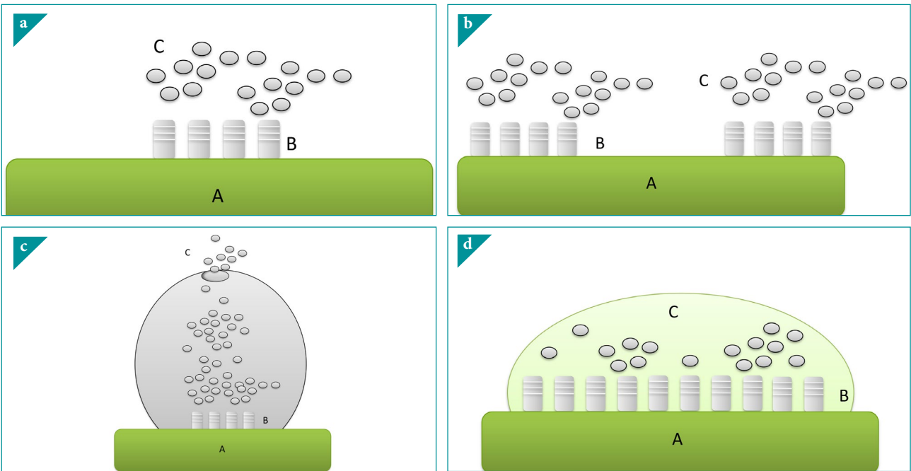
Figura 6.16. Conidios. a. libres, b. en esporodocios, c. en picnidio, d. en acérvulo. A= hospedante, B= conidióforo, C= conidios.
