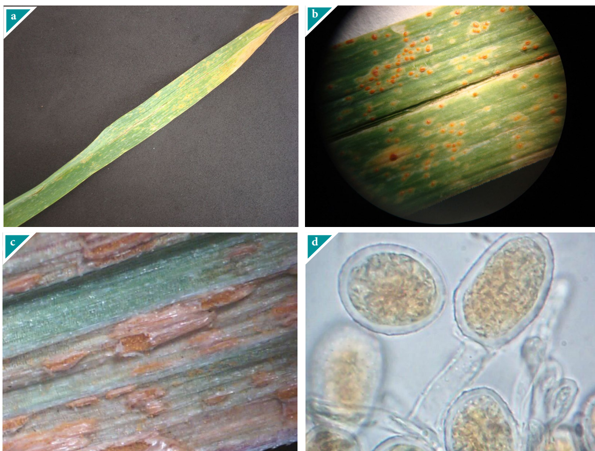
Figura 13.10. Roya anaranjada del trigo, sintomatología: a.b. disposición al azar de las pústulas y la clorosis, c. detalle de pústula, d. urediniosporas.
