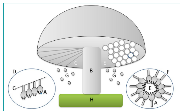
Figura 6.14. Basidiocarpio. Disposición de basidios (A) en laminillas (izquierda) y poros (derecha), B= pie, C= laminillas, D= detalle de laminillas con basidios, E= poros, F= detalle de basidios formando un poro, G= basidiosporas.
