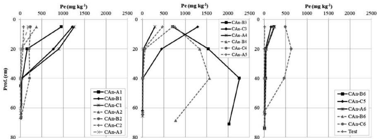
Figura 7. Corral CAn. Concentraciones de Pe en función de la profundidad para los distintos sitios de muestreo del corral.
