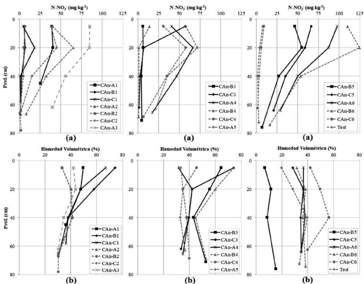
Figura 6. Corral CA. Concentraciones de N-NO_3^- y contenido de humedad volumétrica en función de la profundidad para los distintos sitios de muestreo.
