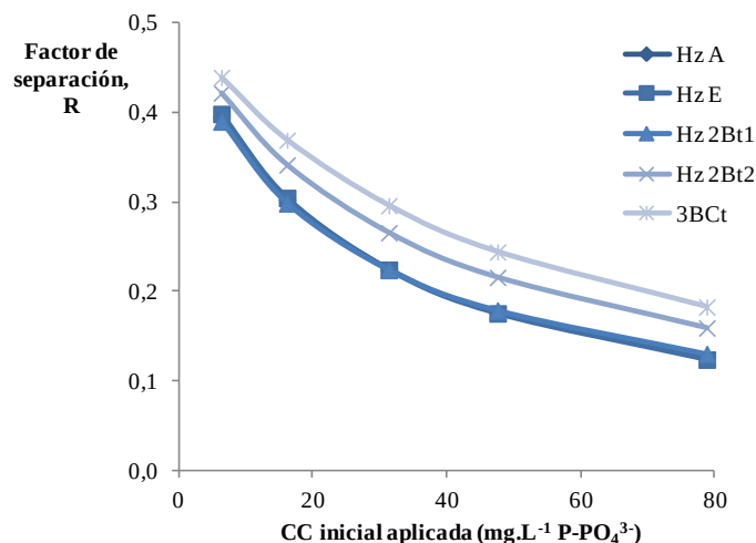
Fig. 2: Factor R medio para cada horizonte en función de las concentraciones aplicadas de P. Hz.: Horizonte. n_{\text{Hz A}} = 45 ; n_{\text{Hz E}} = 15 ; n_{\text{Hz Bt1}} = 45 ; n_{\text{Hz Bt2}} = 35 ; n_{\text{Hz BCt}} = 10 .
