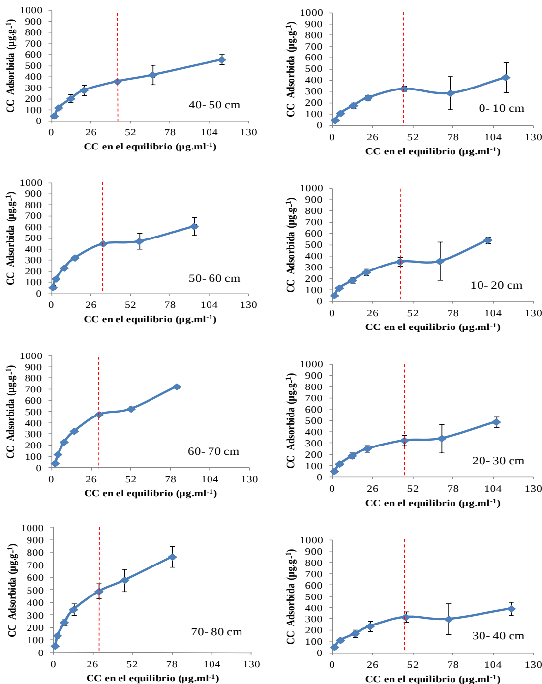
Fig. 1: Isotermas de adsorción de P en el suelo. Línea punteada: punto de la curva de mínima pendiente de la recta tangente. CC: Concentración.
