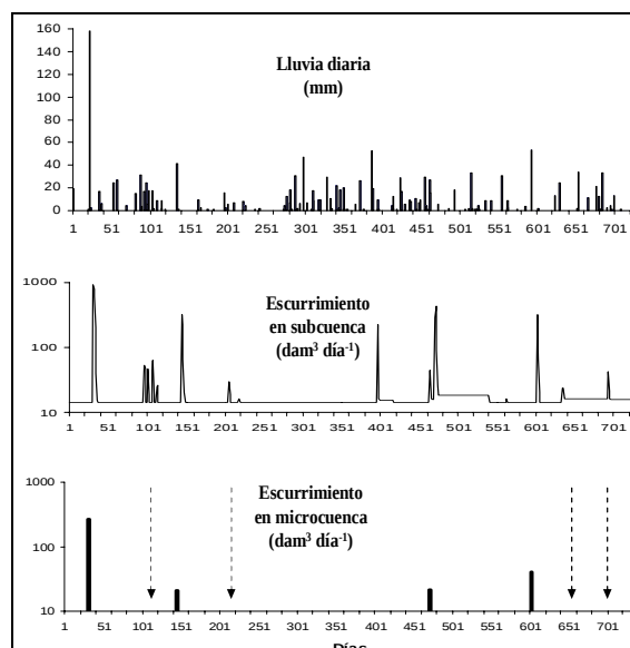
Figura 3. Lluvias y escurrimientos directos diarios registrados en el Arroyo del Tala a nivel de subcuenca (409 km 2 ) y de microcuenca (3 km 2 ). Las líneas verticales punteadas indican los eventos de escurrimiento directo producidos en la subcuenca que no tuvieron su correlato en la microcuenca. Período 2004-2005 (adaptado de Chagas, 2007).
