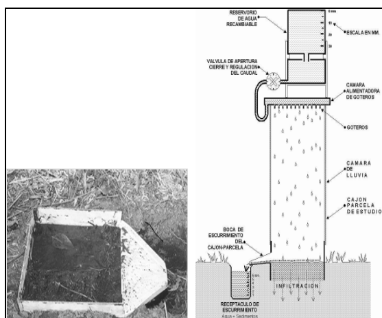
Figura 4. Esquema del simulador de lluvias y detalle del bastidor de la microparcela de escurrimiento, clavado en el suelo (adaptado de Iurtia y Mon, 1994).
