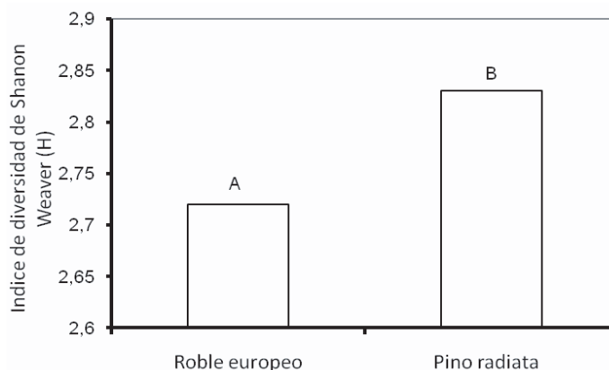
Figura 2. Índice de Shannon-Weaver (H) para las medias de los tratamientos en el suelo bajo la influencia de las especies Roble europeo o eslavonia ( Quercus robur ) y Pino radiata ( Pinus radiata D. Don.). Letras distintas indican diferencias significativas entre especies forestales, mediante tests de Tukey ( \alpha = 0,05 ).
