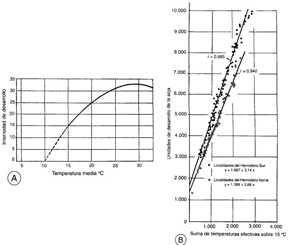
FIGURA 15.3. A) Relación promedio entre la temperatura y la velocidad de desarrollo de la soja. B) Correlación entre Unidades de Desarrollo y suma de temperaturas residuales sobre 15\text{ }^\circ\text{C} .
